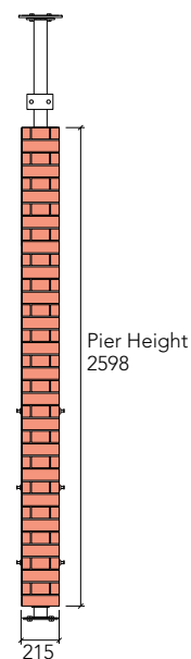
Elevation
